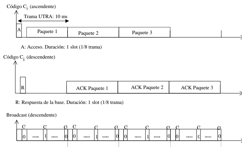
Figura 1. El protocolo ISMA/CDMA
